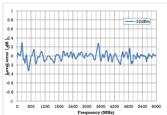
电平误差VS 频率, 输出电平= -32 dBm
