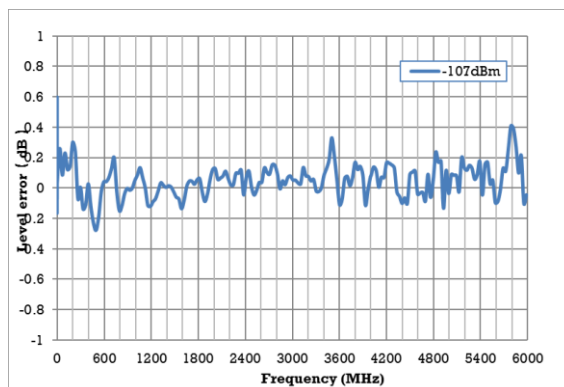
电平误差VS 频率, 输出电平= -107 dBm
